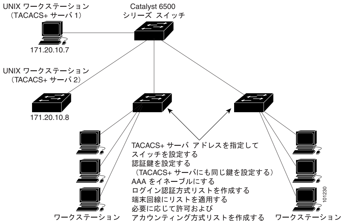
図 8-1 一般的な TACACS+ ネットワーク構成
