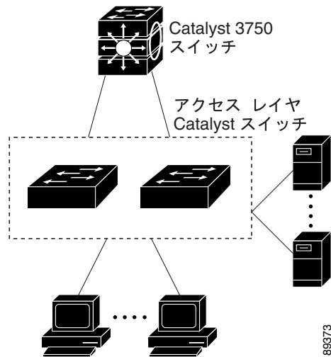
図 1-1 高性能なワークグループ (GHHD)
