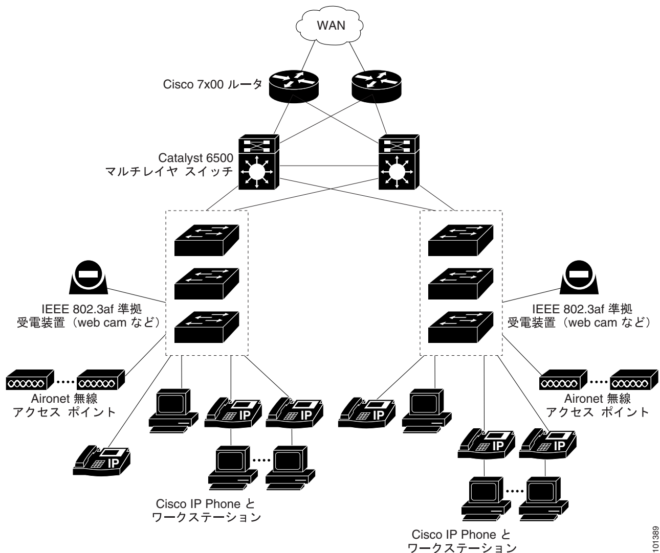
図 1-4 バックボーン構成でのワイヤリングクローゼットの Catalyst 3560 スイッチ
