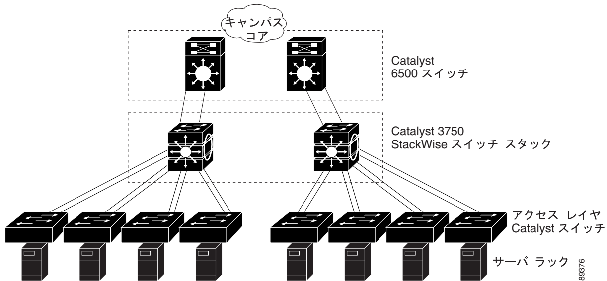
図 1-2 サーバ集約
