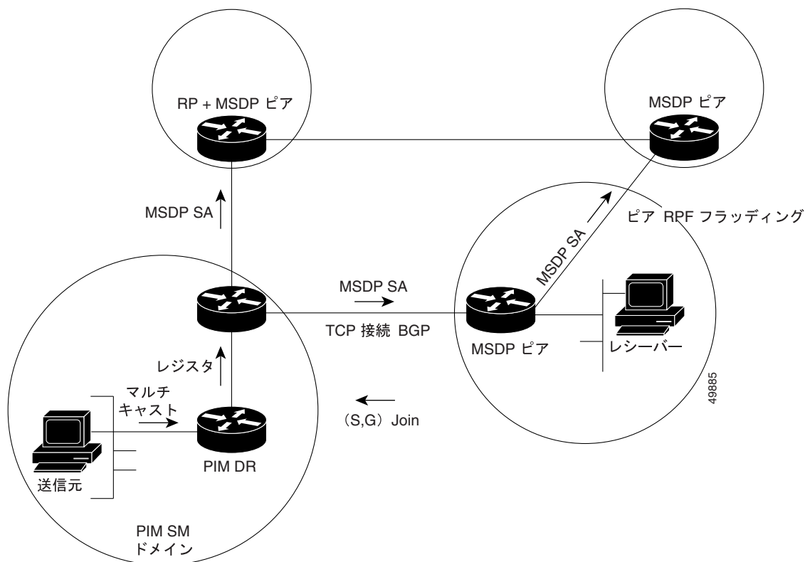
図 36-1 RP ピア間で動作する MSDP
