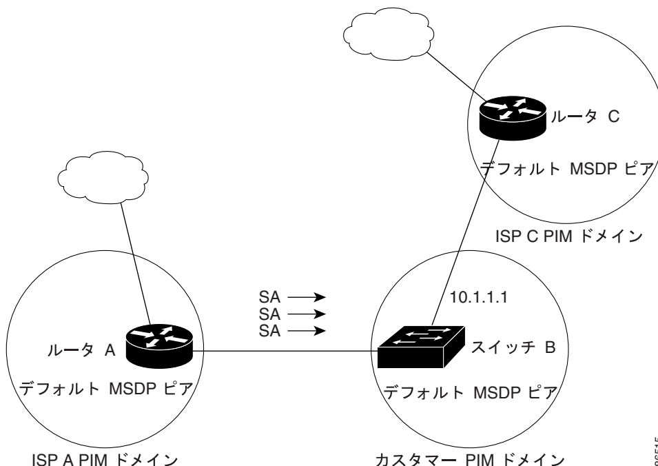
図 36-2 デフォルトの MSDP ピア ネットワーク
