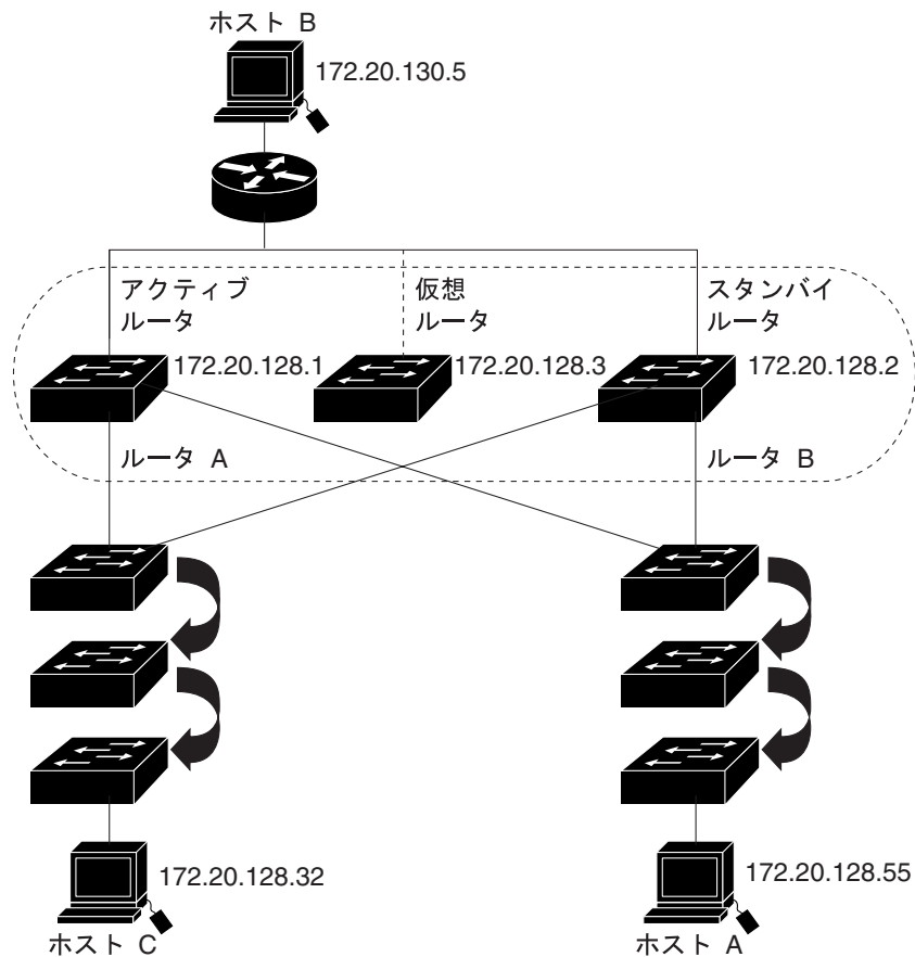
図 33-1 HSRP の一般的な構成
