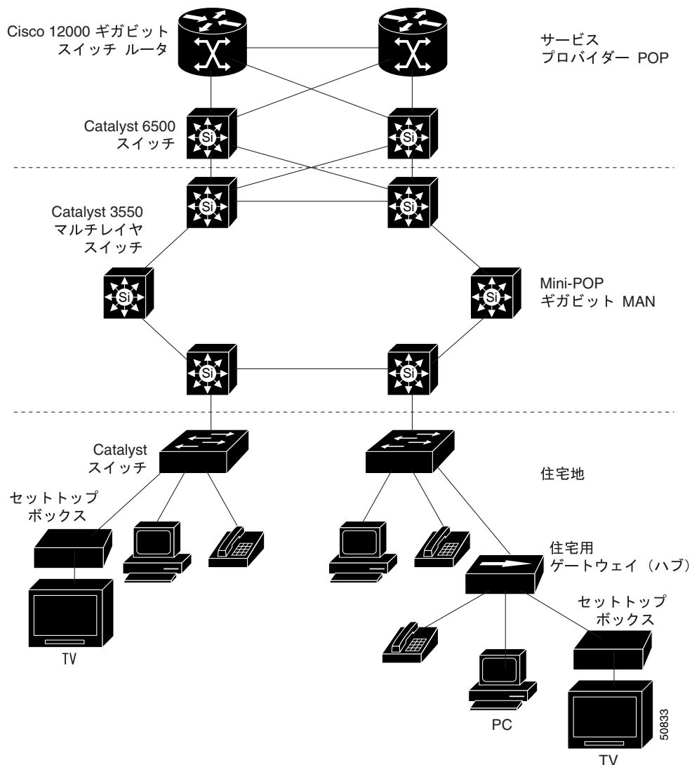
図 1-4 MAN 構成の Catalyst 3550 スイッチ
