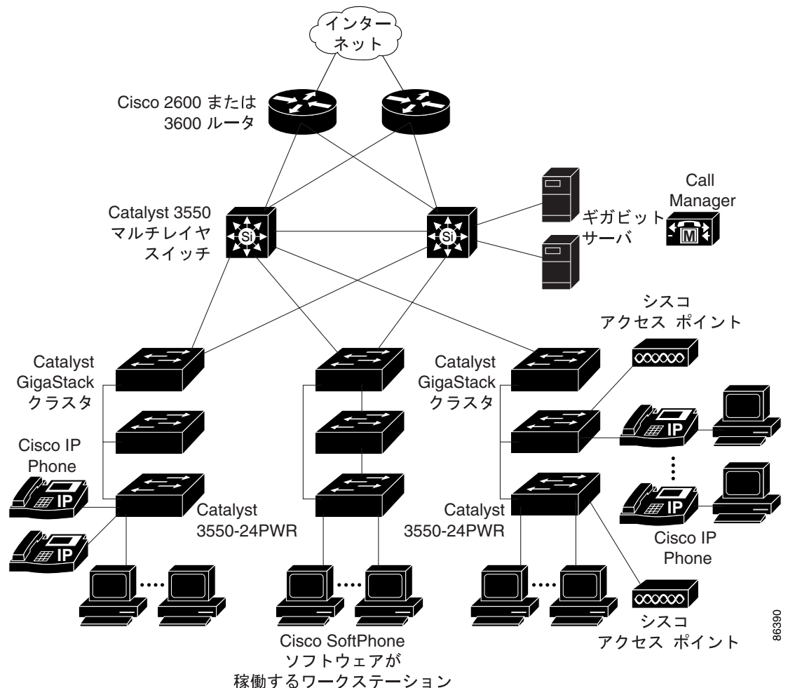
図 1-2 コラプストバックボーン構成の Catalyst 3550 スイッチ
