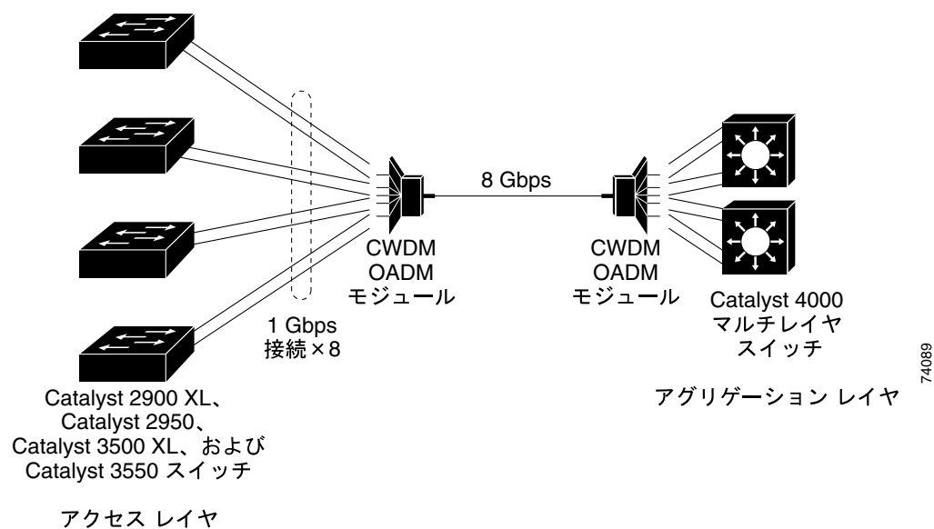
図 1-5 長距離広帯域幅の転送構成
