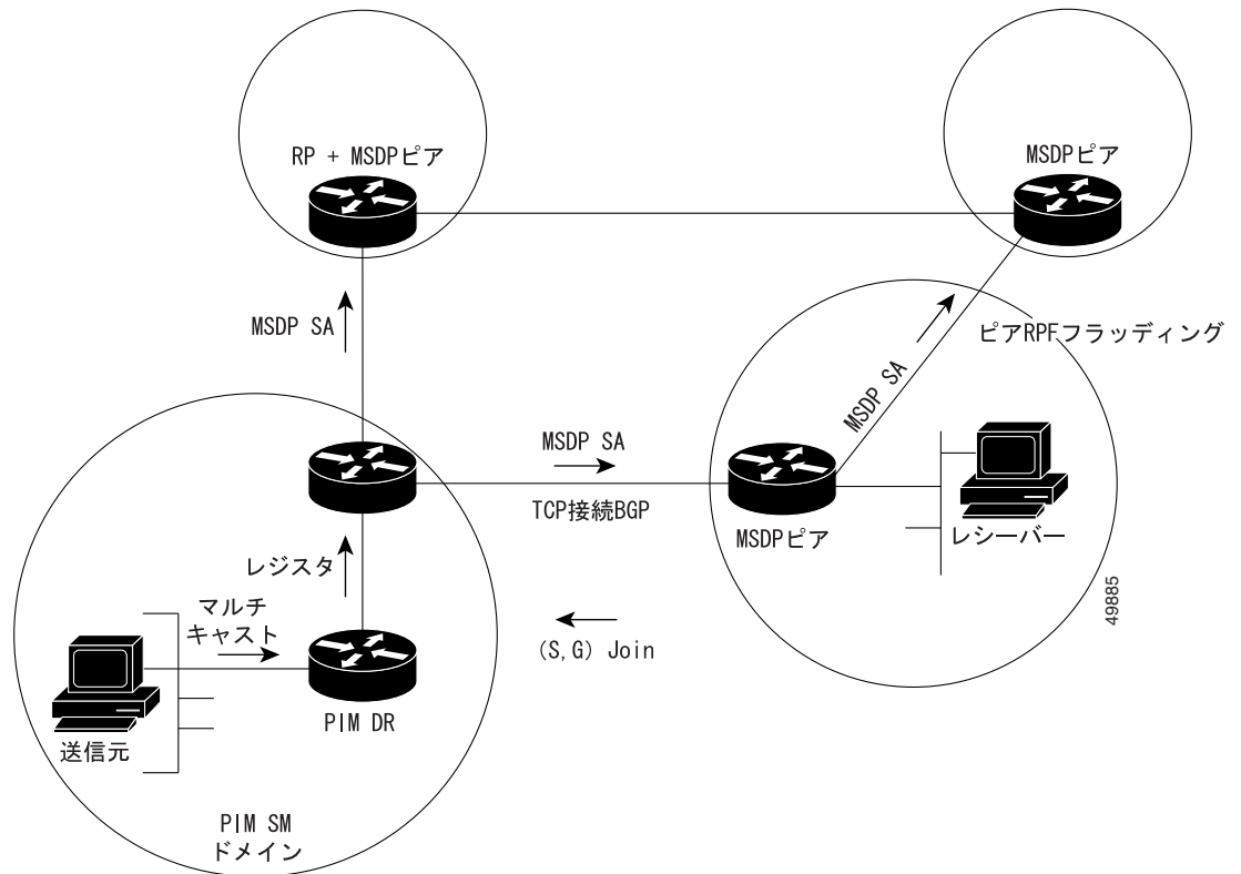
図 35-1 RP ピア間で動作する MSDP
