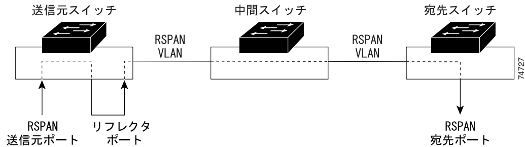
図 24-2 RSPAN 設定の例
