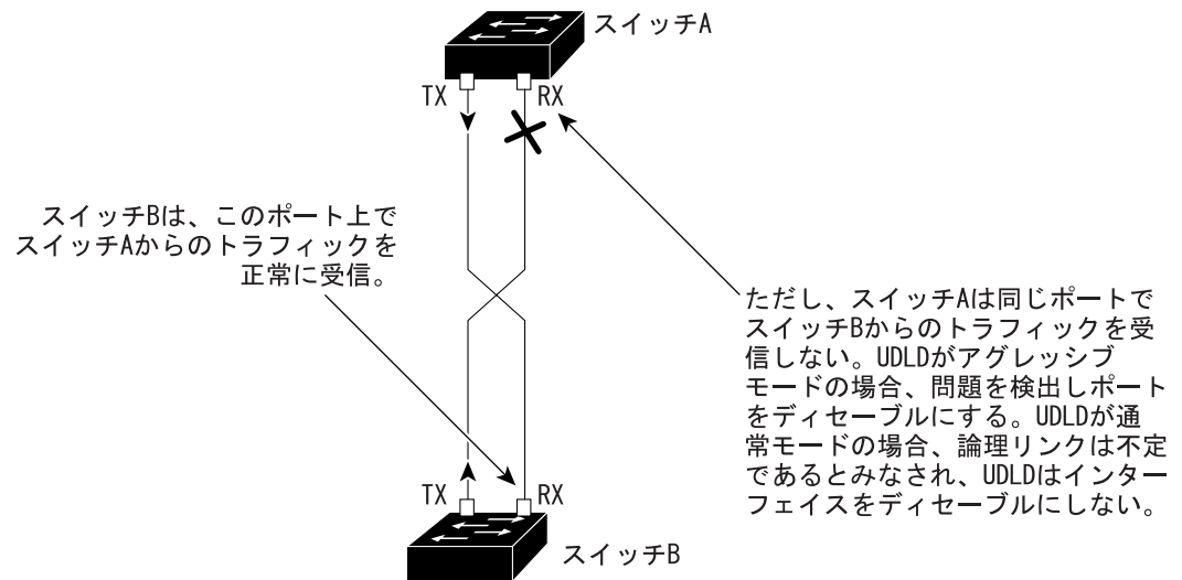
図 23-1 単一方向リンクの UDLD 検出
