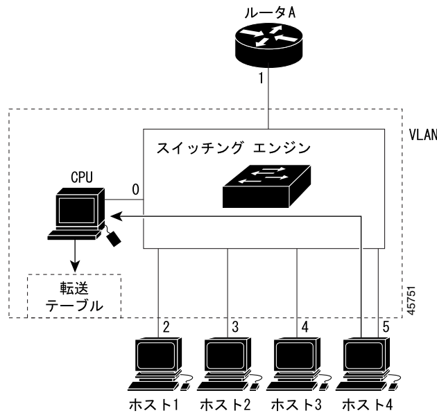
図 20-2 2 番めのホストのマルチキャスト グループへの加入
