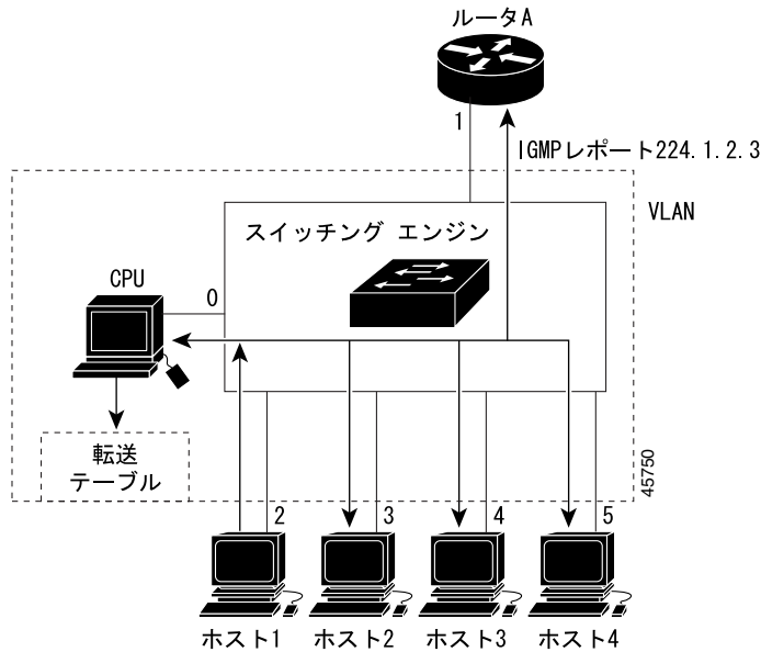
図 20-1 最初の IGMP Join メッセージ
