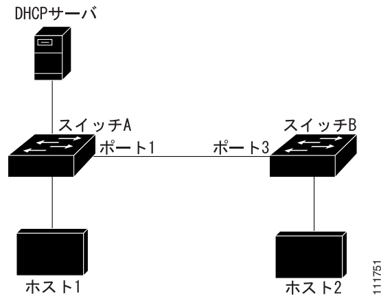
図 19-2 ダイナミック ARP 検査がイネーブ爾である VLAN 上での ARP パケットの検証
