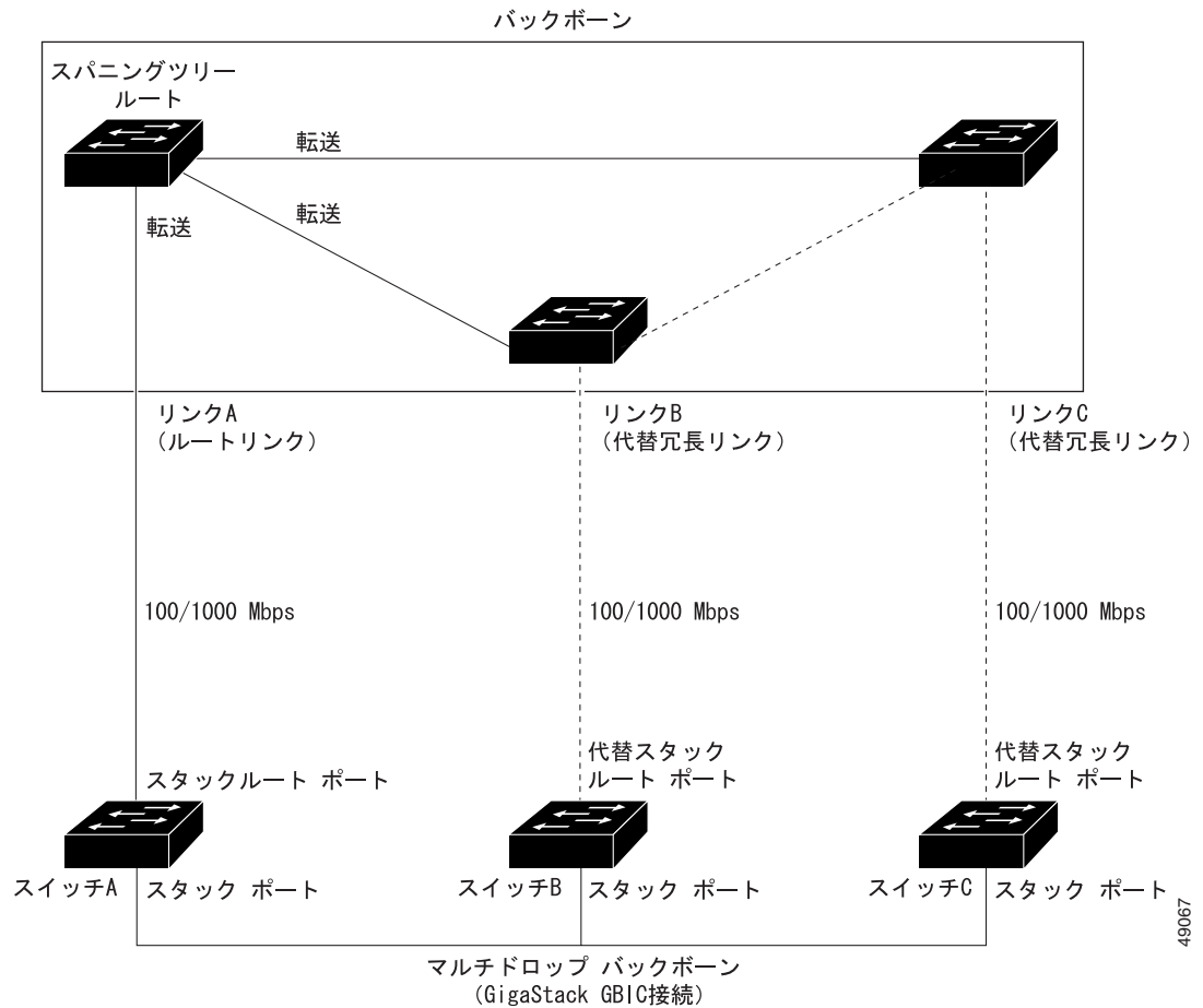
図 17-5 CSUF のトポロジー
