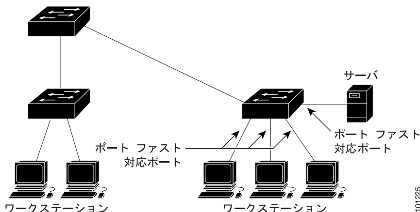
図 17-1 PortFast 対応ポート
