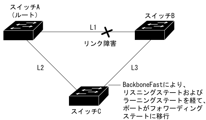
図 17-8 間接リンク障害発生後の BackboneFast の例
