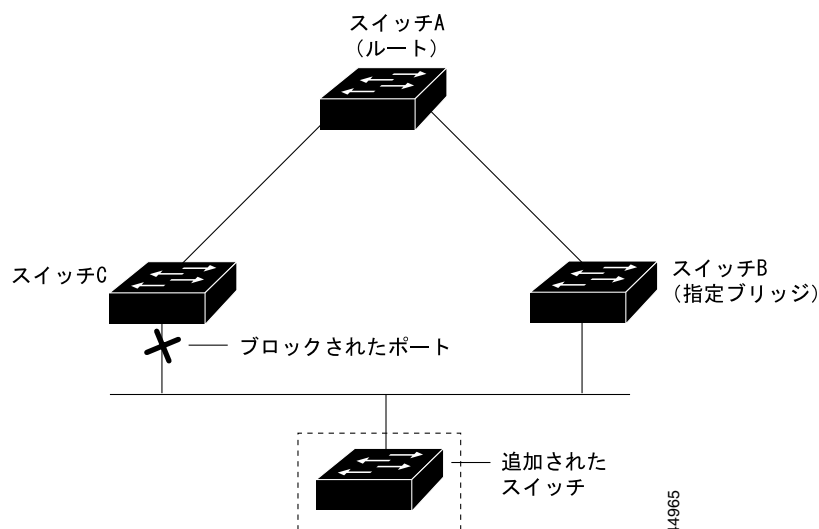
図 17-9 メディア共有型トポロジへのスイッチの追加
