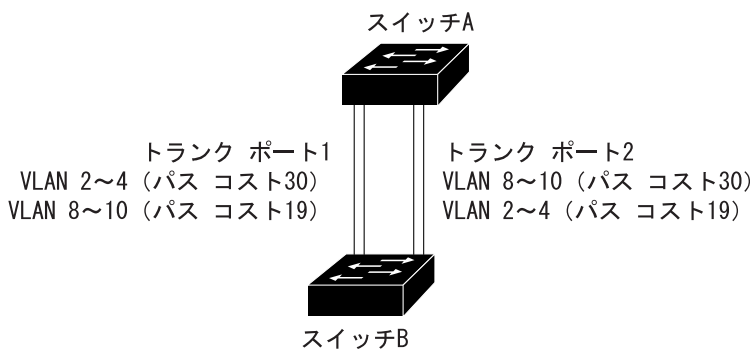
図 11-4 パス コストによってトラフィックが分散されるロード シェアリング トランク
