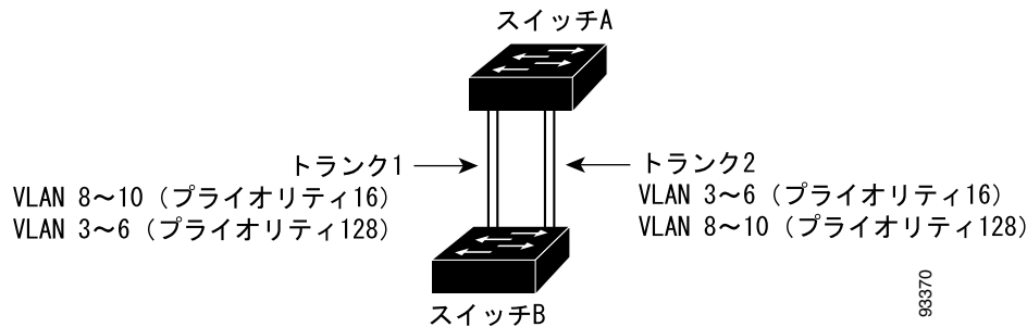
図 11-3 STP ポート プライオリティによるロードシェアリング
