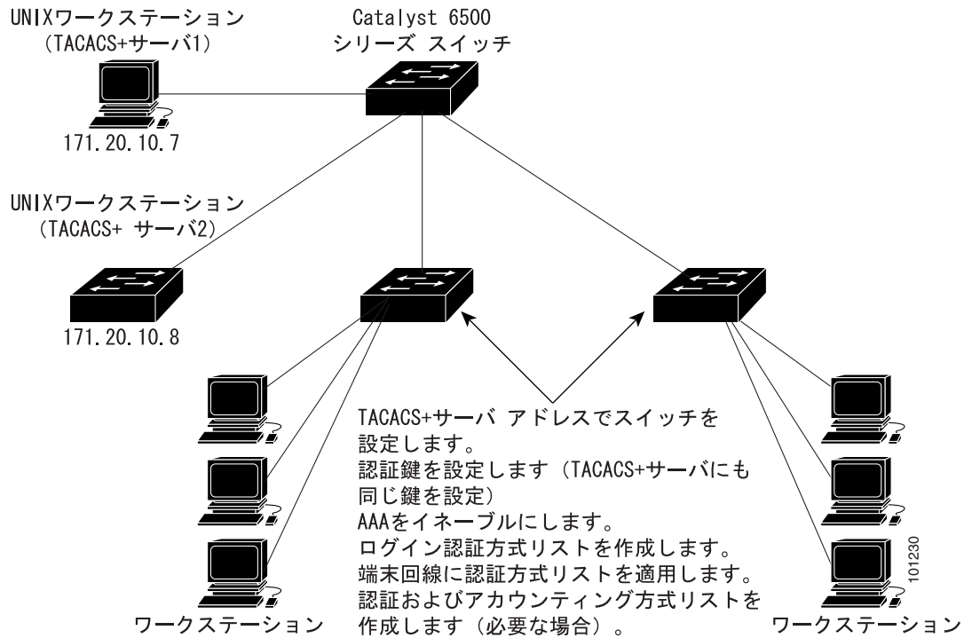
図 7-1 一般的な TACACS+ ネットワーク構成
