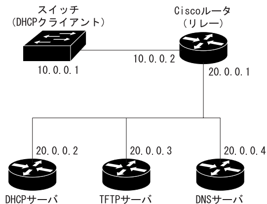
図 3-2 リレー デバイスを使用した自動設定
