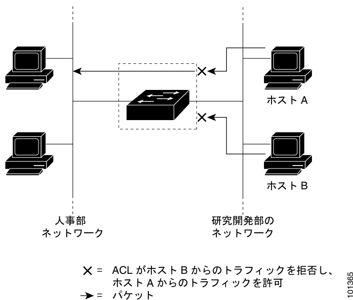
図 28-1 ACL を使用したネットワーク トラフィックの制御
