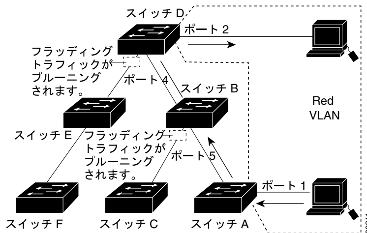
図 13-2 VTP ブルーニングによるフラディングトラフィックの最適化
