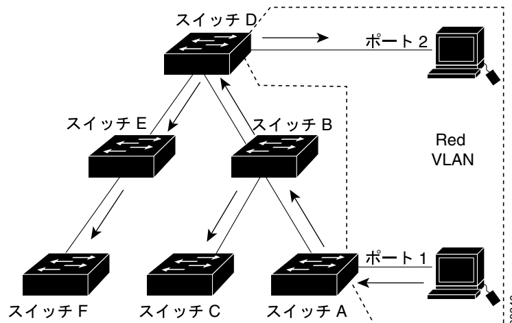
図 13-1 VTP ブルーニングを使用しない場合のフラディングトラフィック
