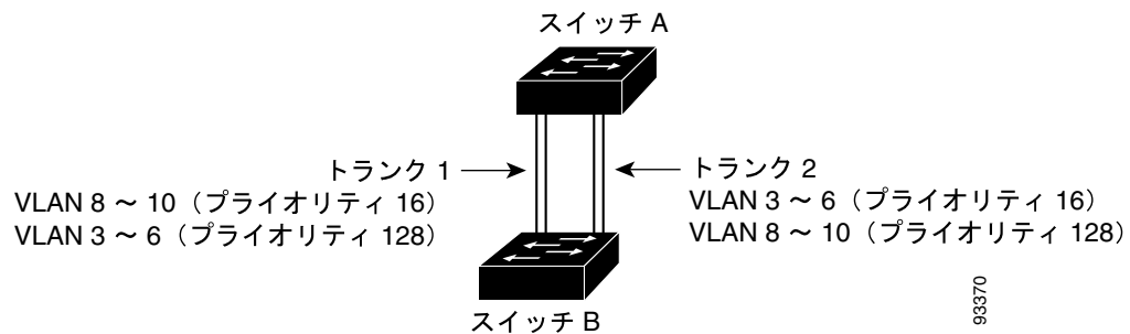
図 12-2 STP ポート プライオリティによる負荷分散
