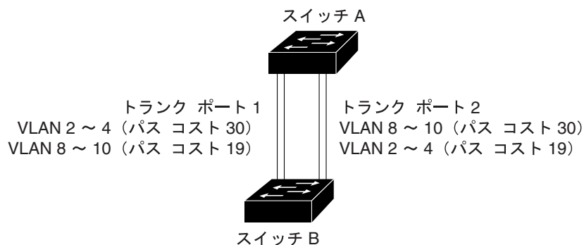
図 12-3 パス コストによってトラフィックが分散される負荷分散トランク
