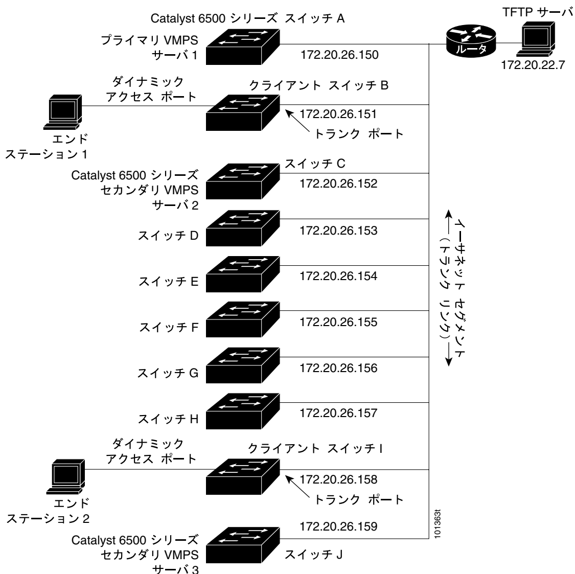
図 12-4 ダイナミック ポート VLAN メンバーシップの構成例
