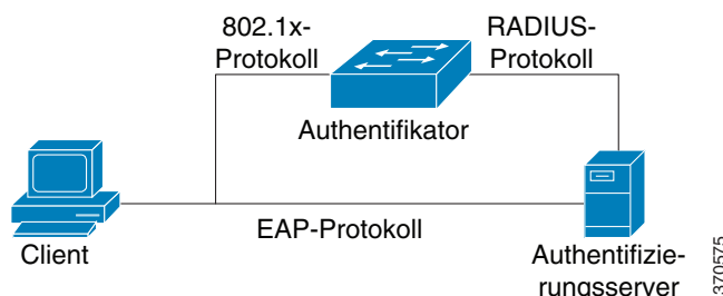
Abbildung 1 802.1X-basierte Authentifizierung
