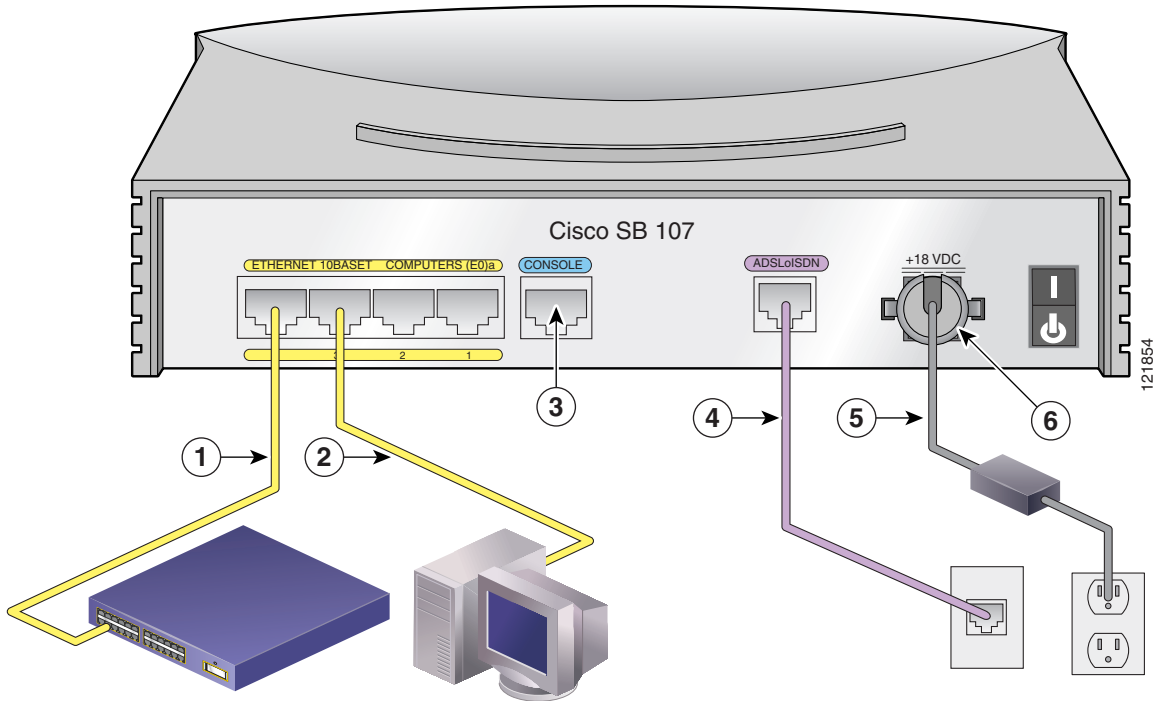
Figura 5-3 Configurazione tipica di Cisco SB 107
