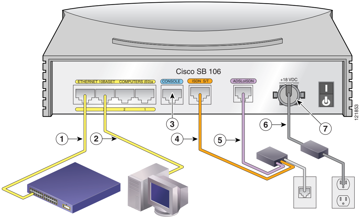
Figura 4-3 Instalación típica de Cisco SB 106
