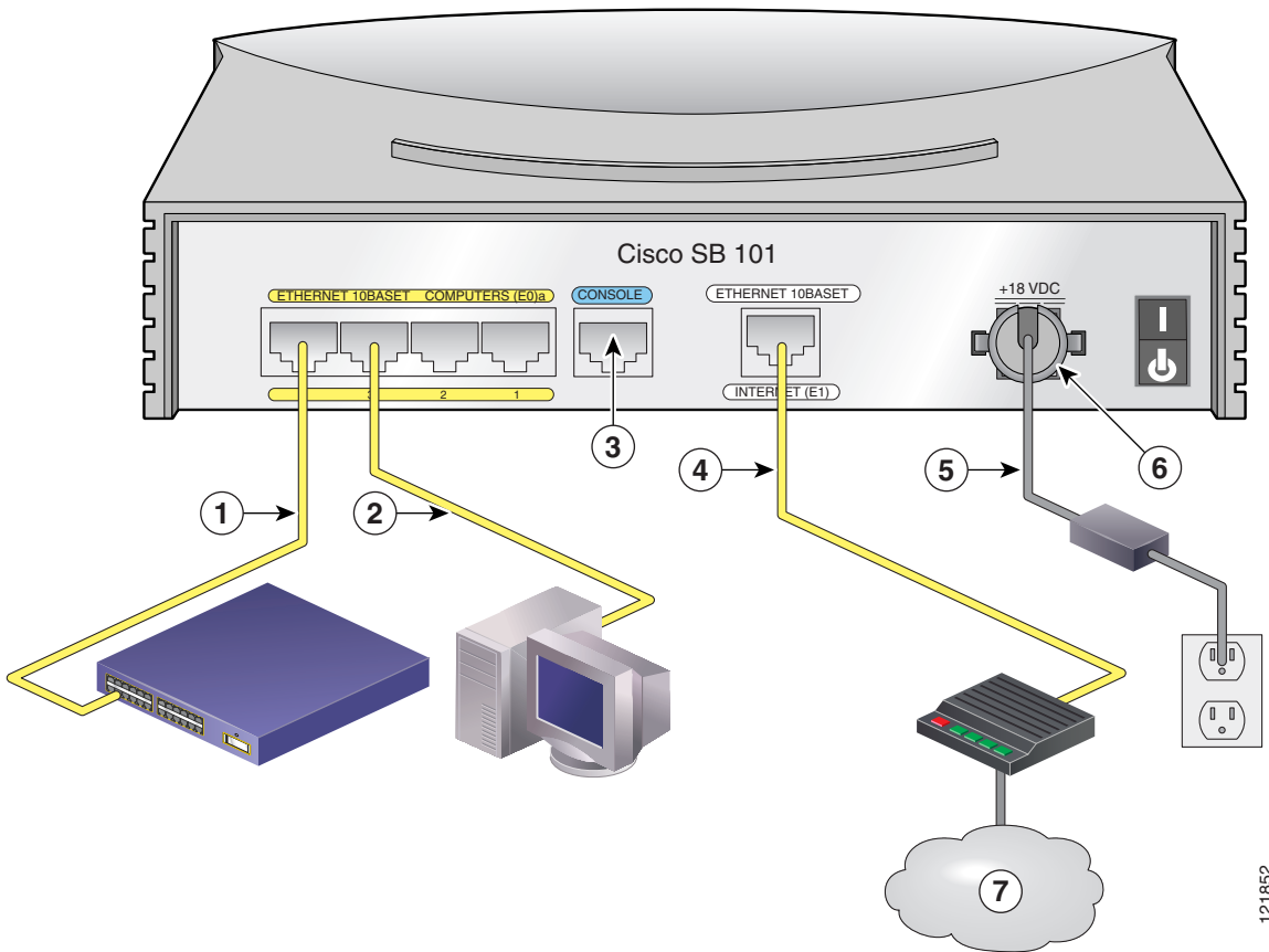
Abbildung 2-3 Typische Cisco SB 101-Installation
