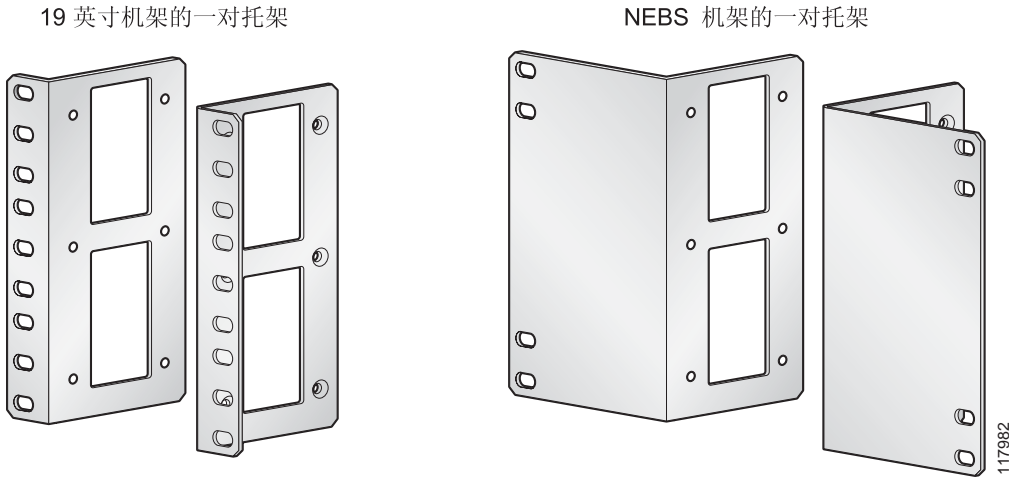
图 4 Cisco 3845 路由器的架式安装托架
