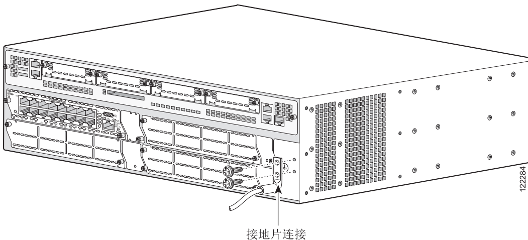
图 11 Cisco 3845 机箱符合 NEBS 标准的机箱接地连接
