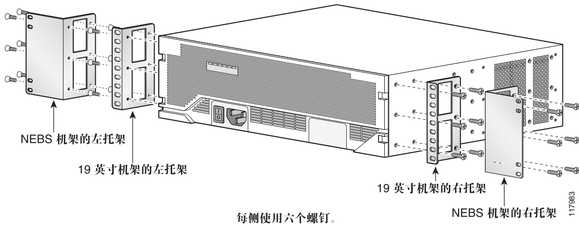
图 5 前面安装模式下的托架安装
