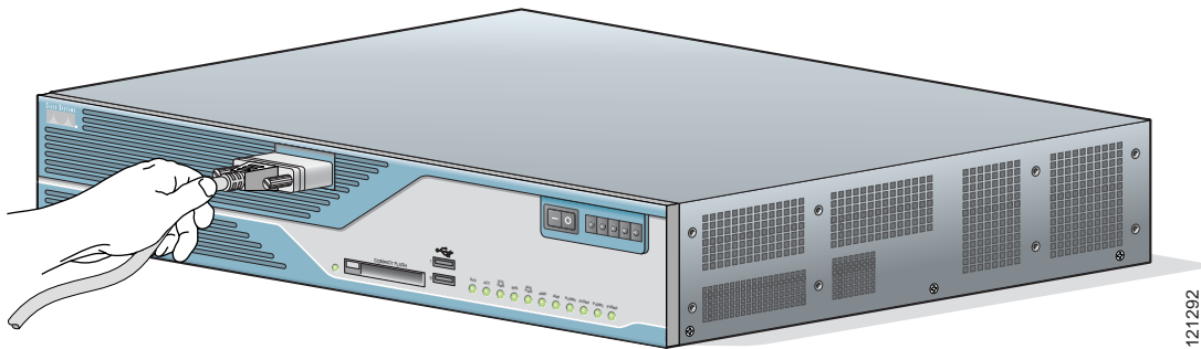
图 17 将 RPS 连接器插到 Cisco 3825 路由器中
