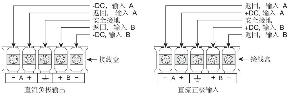
图 12 Cisco 3825 路由器的直流电源连接 (标准)
