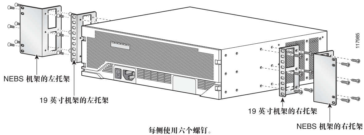
图 7 中心安装模式下的托架安装（前面板朝前）
