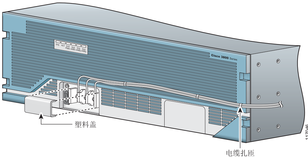
图 15 直流电线布线和连接 (Cisco 3845 路由器)
