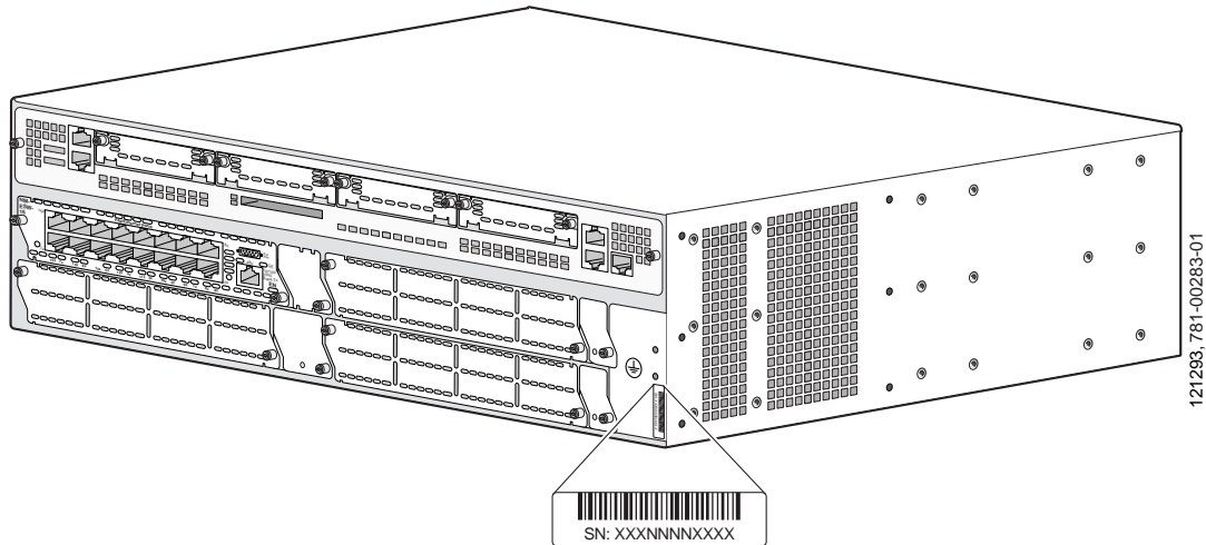
图 2 Cisco 3845 路由器序列号的位置
