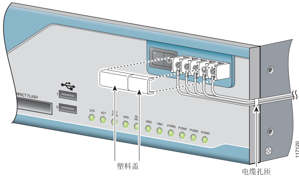
图 14 直流电线布线和连接 (Cisco 3825 路由器)
