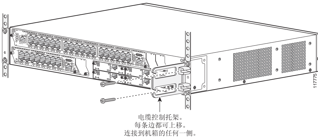
图 9 将电缆管理托架装到 Cisco 3825 路由器上
