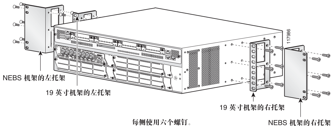
图 8 中心安装模式下的托架安装（后面板朝前）
