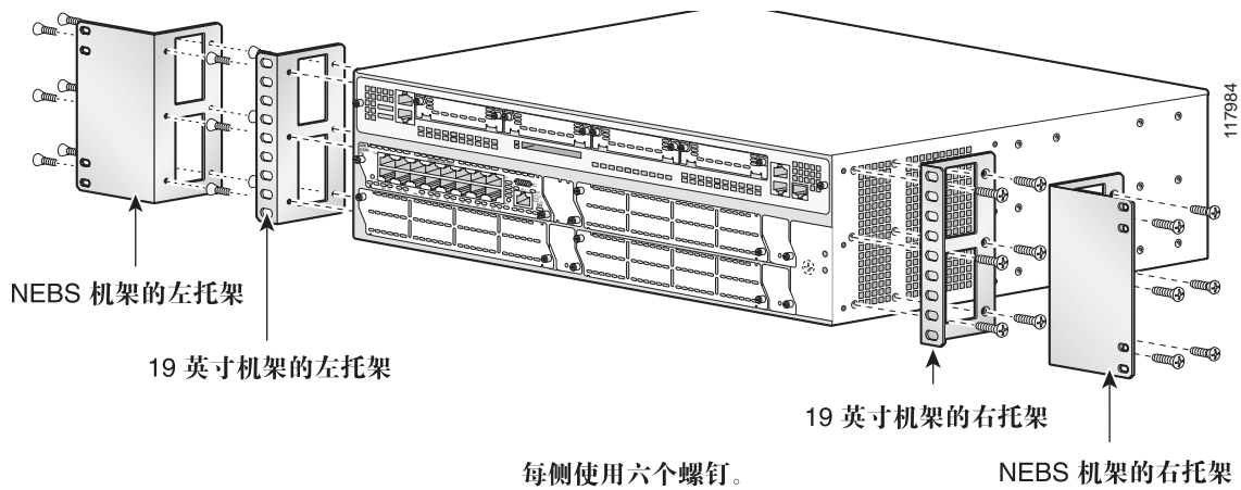
图 6 后面安装模式下的托架安装
