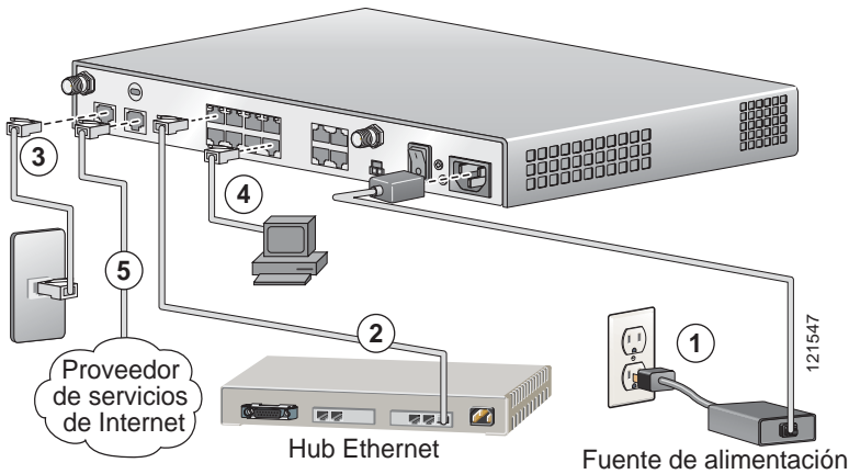
Figura 2 Instalación típica de un router Cisco 1801, Cisco 1802 o Cisco 1803.
