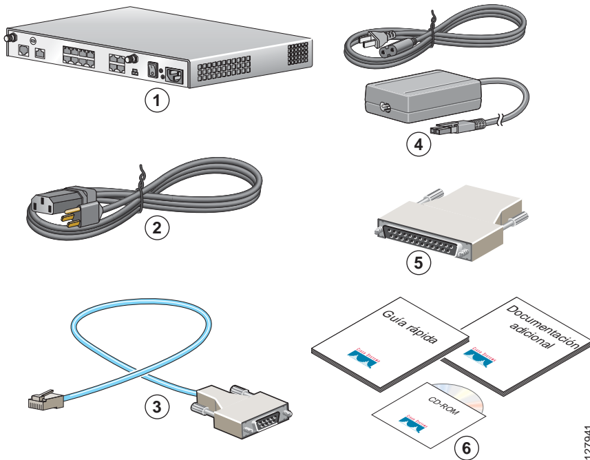
Figura 1 Elementos incluidos con los routers Cisco 1801, Cisco 1802 y Cisco 1803 de servicios integrados
