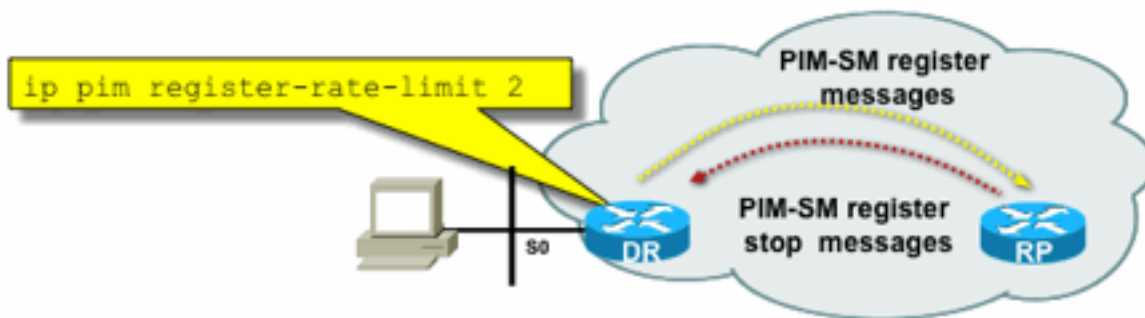
Figura 8: Controle de túnel de registro PIM-SM
