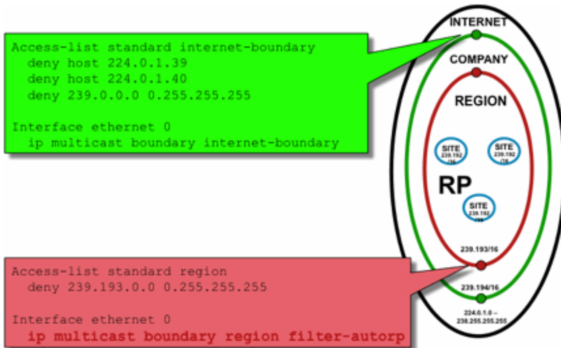
Figura 12: Filtros/escopos de RP automático
