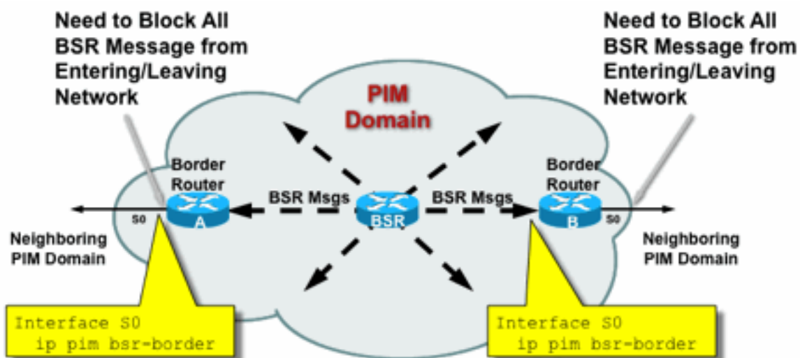
Figura 11: Borda BSR
