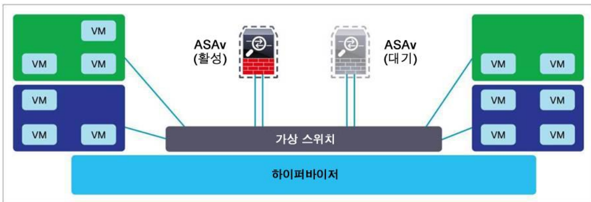
그림 1. ASAv 아키텍처
