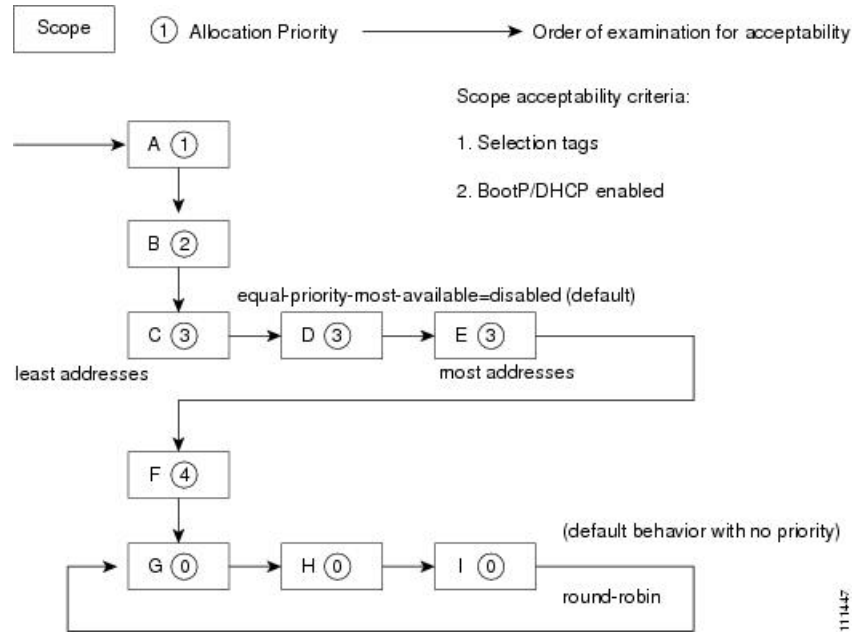
図 11: スコープ割り当て優先順位
