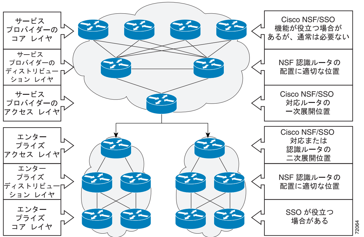
図 5-2 Cisco NSF/SSO ネットワーク展開：エンタープライズ ネットワーク
