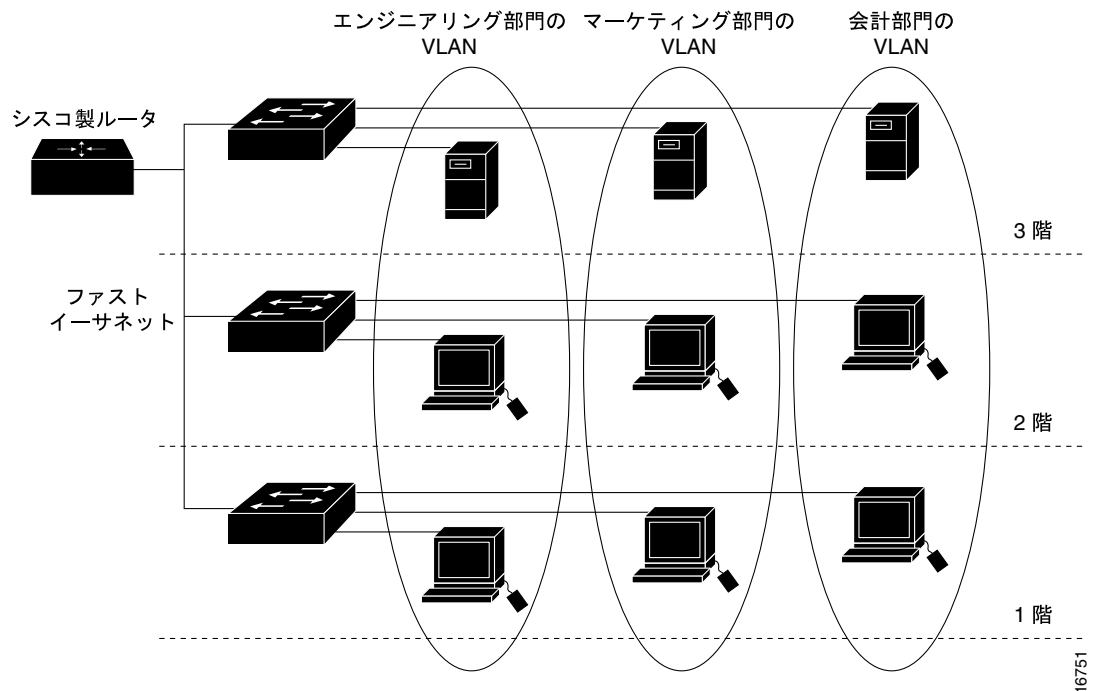
図 13-1 VLAN の例
