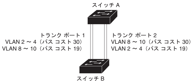
図 16-4 パス コストによってトラフィックが分散される負荷分散トランク
