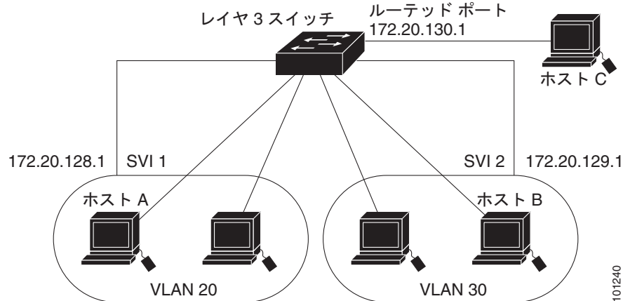
図 54-1 フォールバックブリッジングネットワークの例
