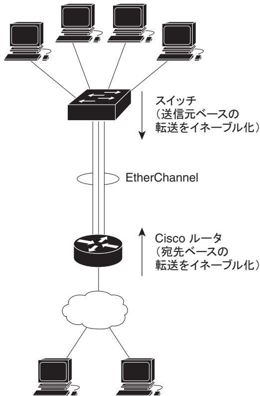
図 42-5 負荷の分散および転送方式
