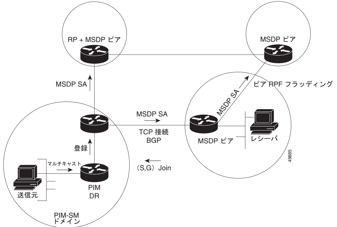
図 48-1 RP ピア間で動作する MSDP
