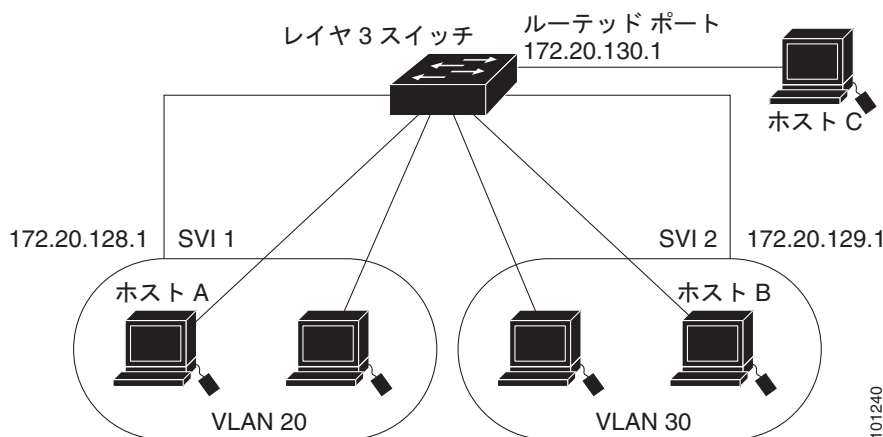
図 49-1 フォールバックブリッジングネットワークの例
