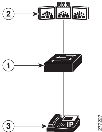
図 38-2 電話機 - スイッチ - コーデック接続
