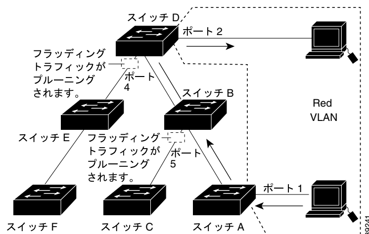
図 17-2 VTP プルーニングによるフラッドイング トラフィックの最適化
