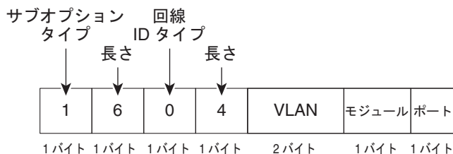
図 26-2 サブオプションのパケット形式
