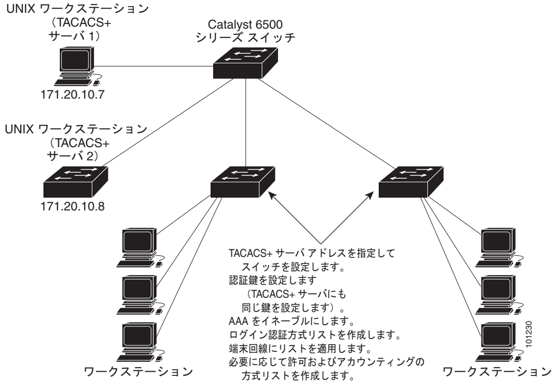
図 11-1 一般的な TACACS+ ネットワーク構成
