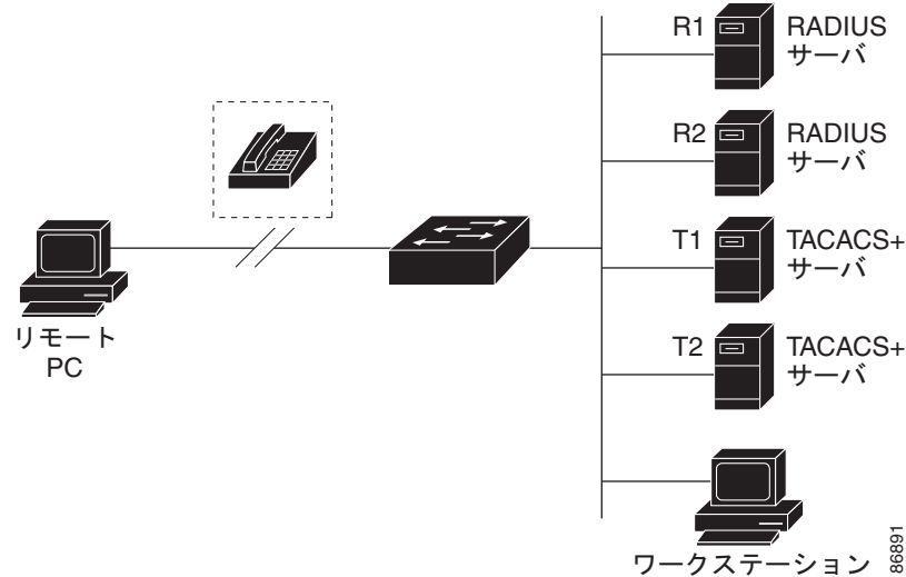
図 11-2 RADIUS サービスから TACACS+ サービスへの移行
