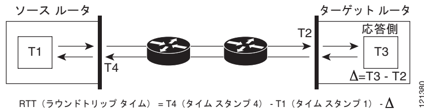
図 67-2 Cisco IOS IP SLA Responder タイムスタンプ
