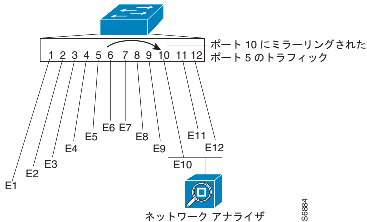
図 56-1 SPAN の設定例
