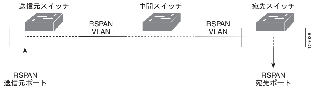
図 56-2 RSPAN の設定例
