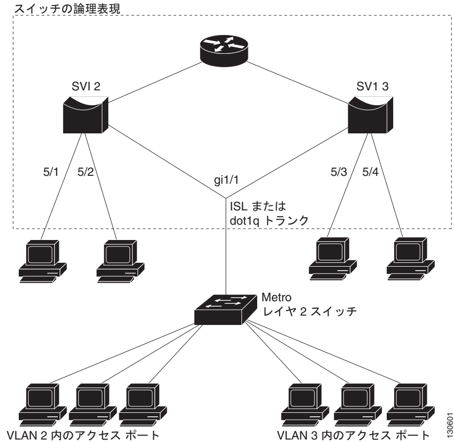
図 48-2 トランク ポート セキュリティ
