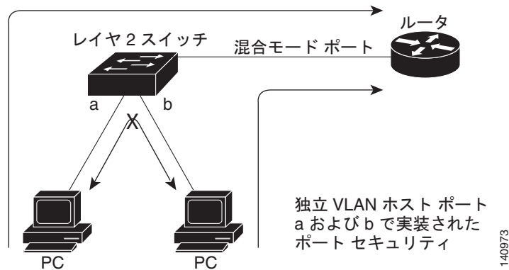
図 48-1 独立 PVLAN ホスト ポートのポートセキュリティ
