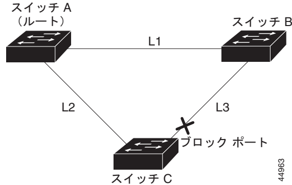
図 20-6 間接リンク障害が発生する前の BackboneFast の例
