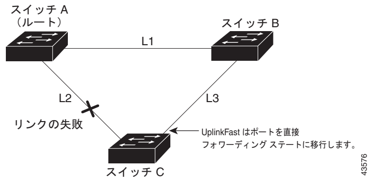
図 20-4 直接リンク障害が発生した後の UplinkFast の例
