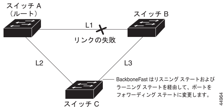
図 20-7 間接リンク障害が発生した後の BackboneFast の例
