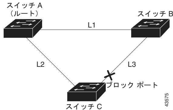
図 20-3 直接リンク障害が発生する前の UplinkFast の例
