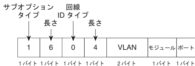
図 22-2 サブオプションの packets 形式
