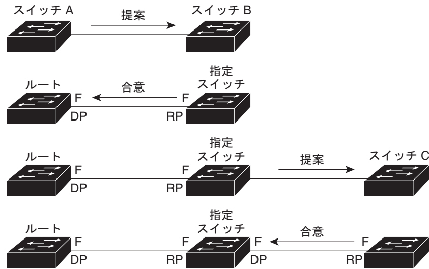
図 21-4 高速コンバージェンスの提案と合意のハンドシェーク
