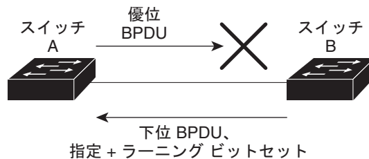
図 21-3 単一方向リンク障害の検出
