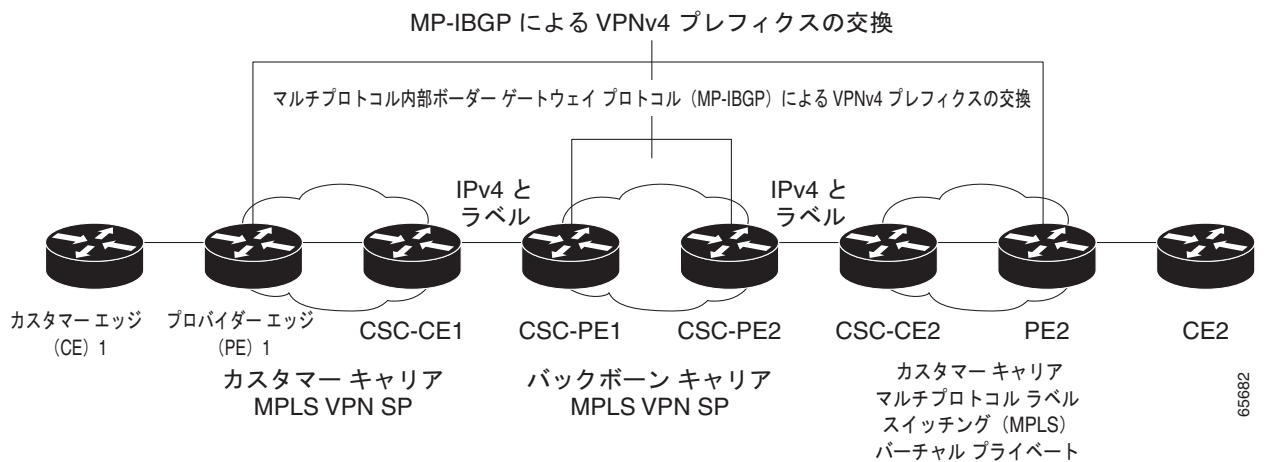
図 5 ネットワーク：カスタマー キャリアが MPLS VPN サービス プロバイダー
