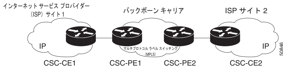
図 4 ネットワーク：カスタマー キャリアが ISP
