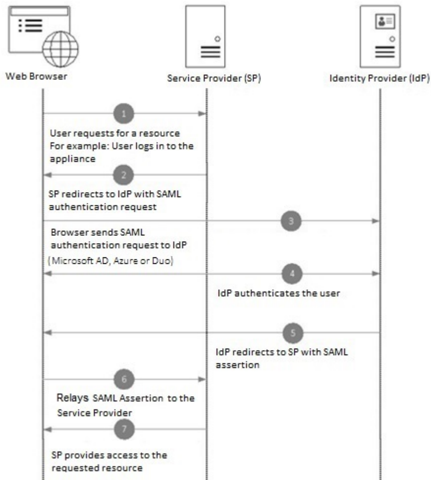
图 3: SAML 工作流
