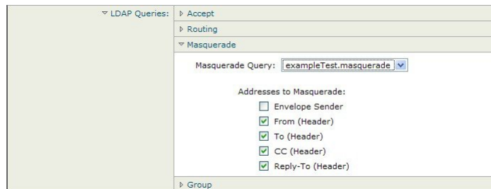
Figure 64: 在侦听程序上启用伪装查询
