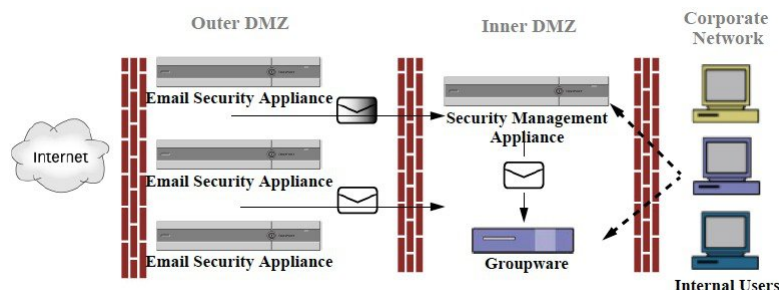
Figure 91: 利用思科安全邮件和 Web 管理器的典型网络配置
