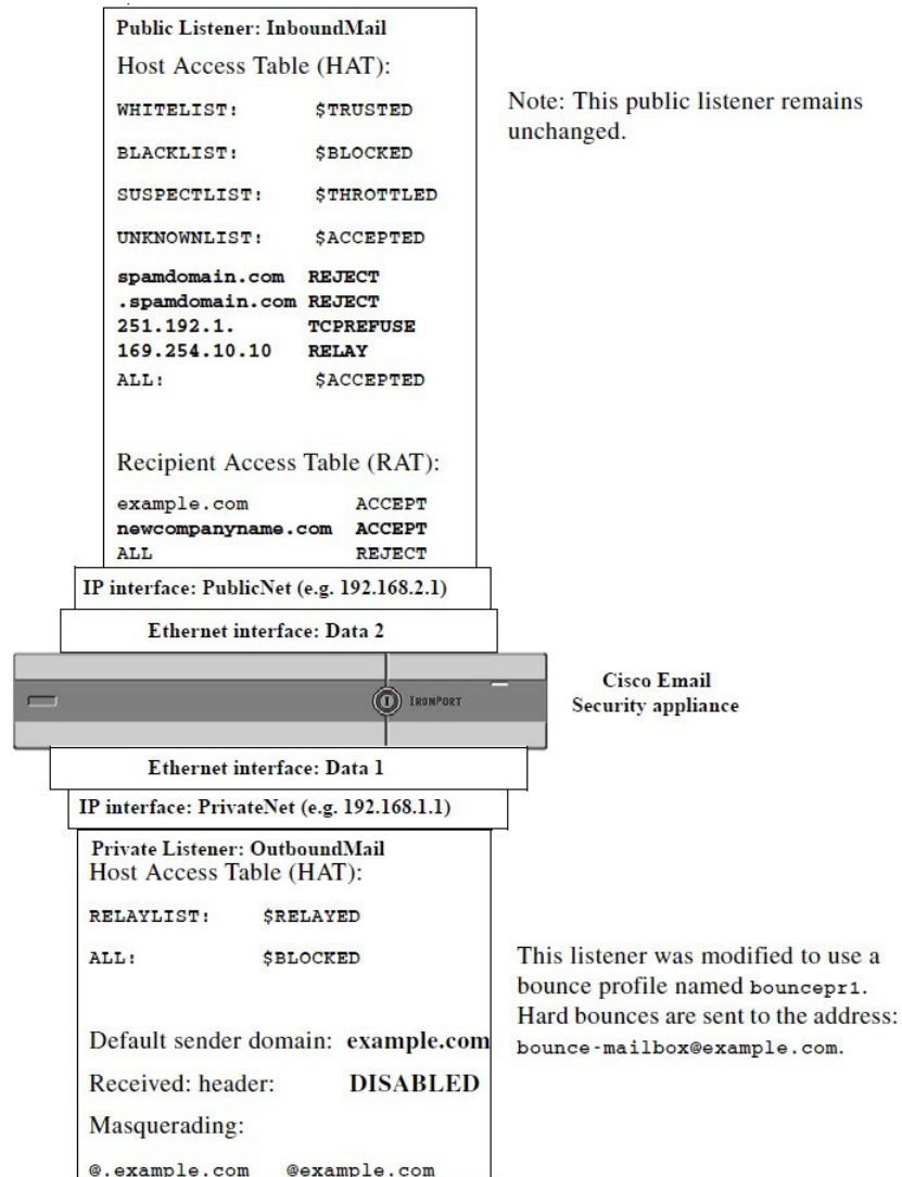
Figure 52: 将退回配置文件应用到专用侦听程序
