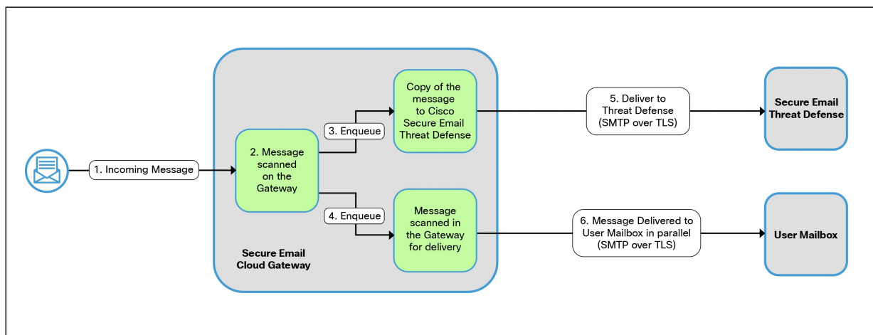
图 19: 威胁防御连接器概述
