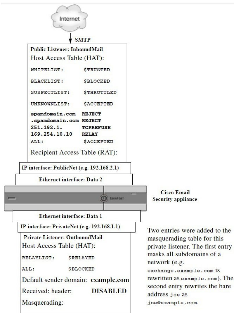
Figure 50: 为专用侦听程序定义的伪装
