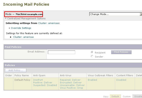
Figure 83: GUI 中的集中管理功能：未定义设置
