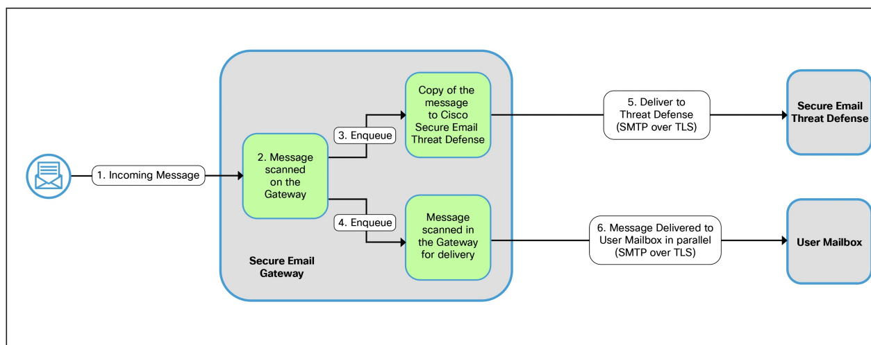
图 19: 威胁防御连接器概述
