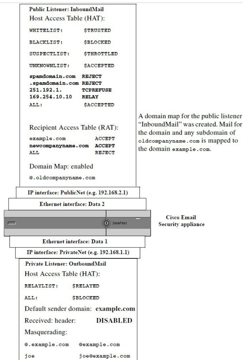
Figure 51: 为公共侦听程序定义的域映射
