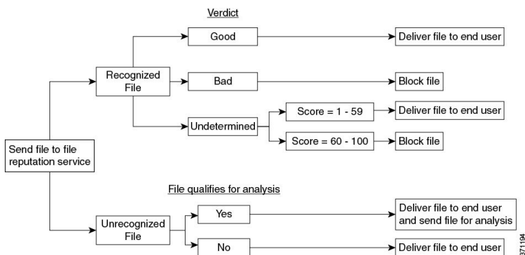
Figure 35: 面向公共云文件分析部署的思科高级恶意软件保护 工作流程
