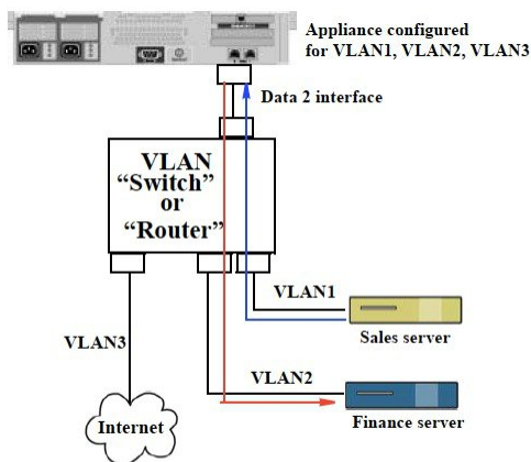
Figure 79: 使用 VLAN 加速邮件网关之间的通信
