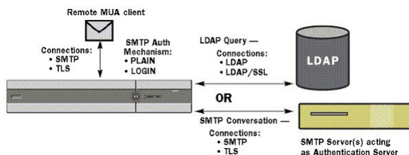
Figure 68: SMTP Auth 支持: LDAP 目录存储或 SMTP 服务器
