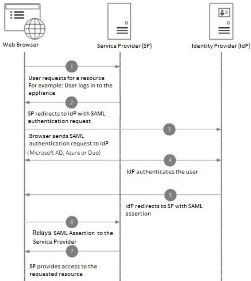
图 78: SAML 工作流程
