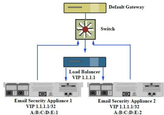
Figure 80: 使用 DSR 实现交换机上多个邮件网关之间的负载均衡
