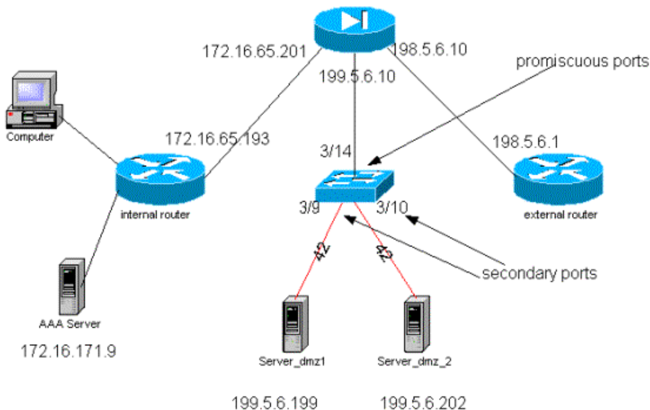
Figura 5: Ambiente de Teste da DMZ Externa
