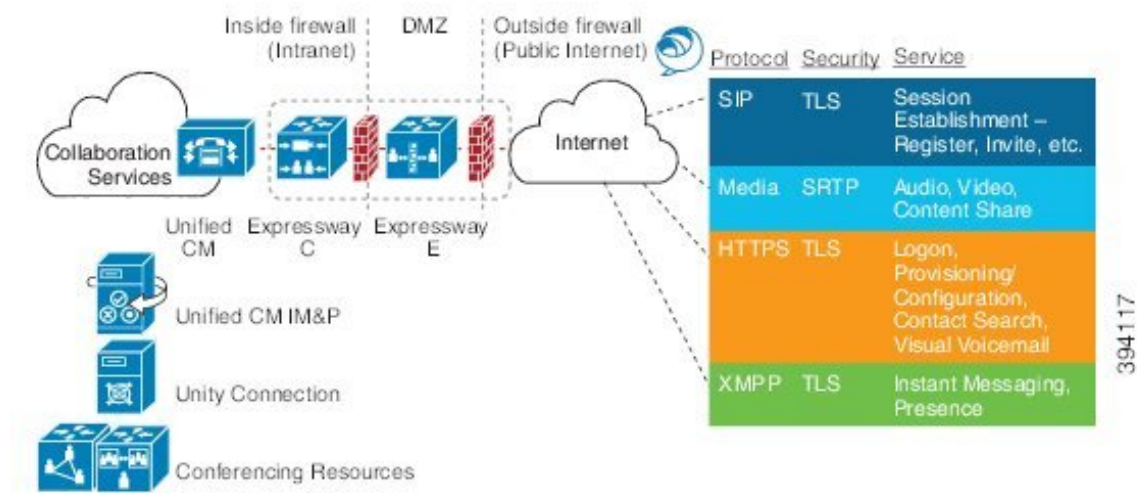
図 3: プロトコルワークロード概要
