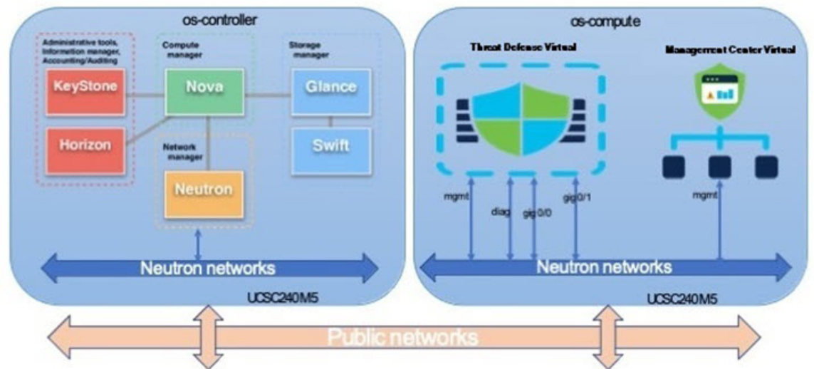
図 49: OpenStack で Threat Defense Virtual と Management Center Virtual を使用したトポロジの例
