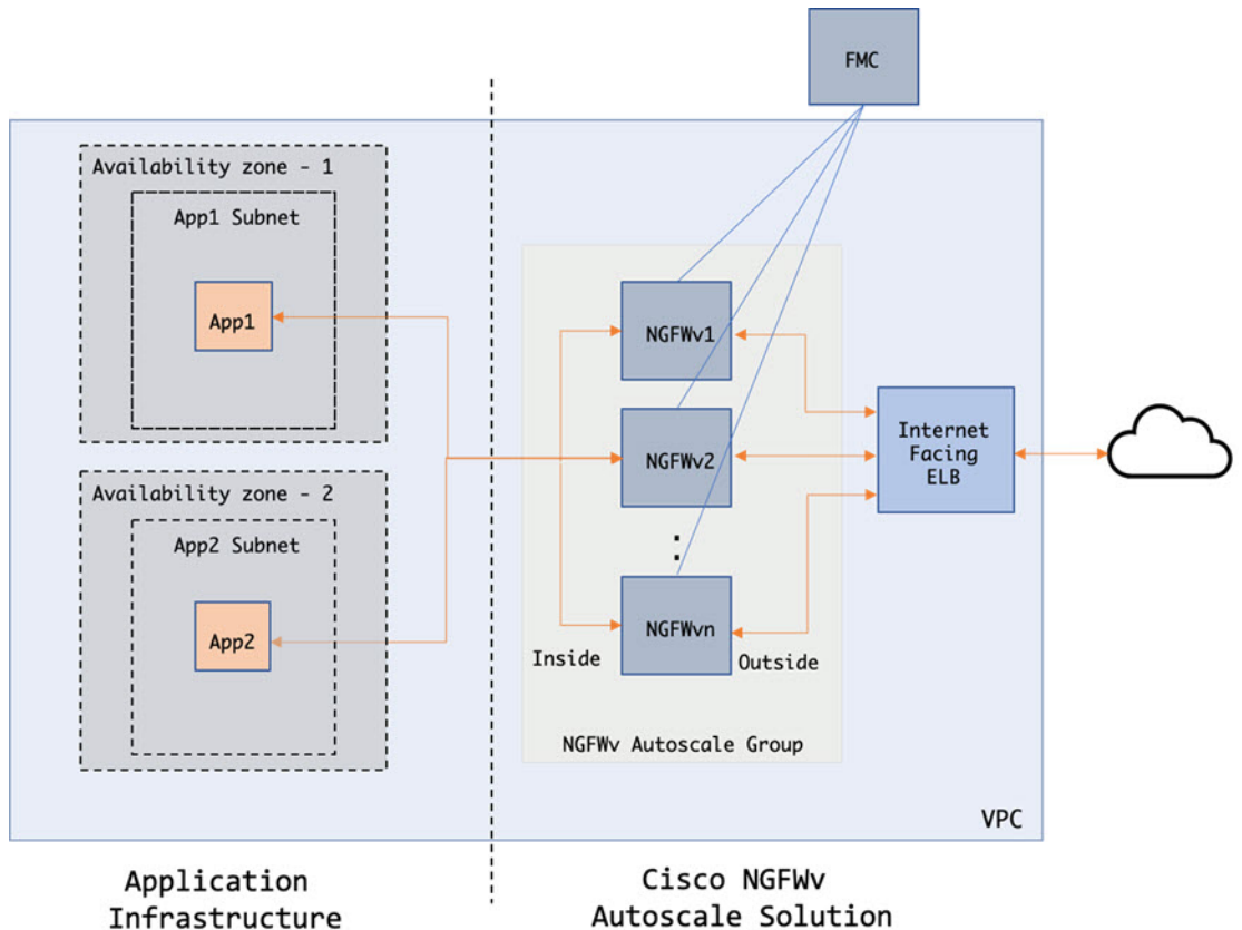
図 3: Threat Defense Virtual Auto Scale の導入例の図
