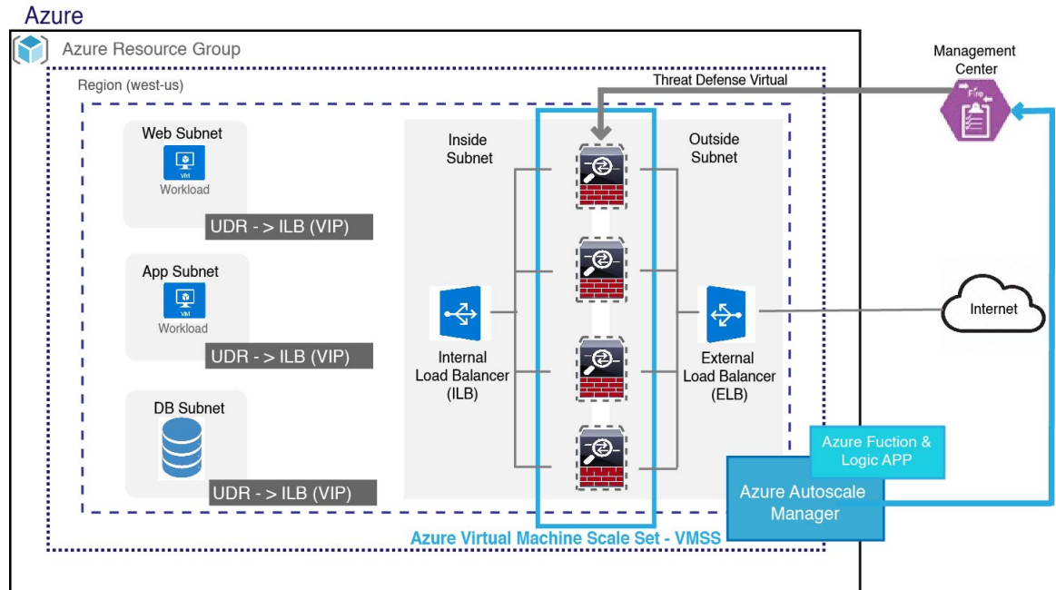
図 5: サンドイッチトポロジを使用した Threat Defense Virtual Auto Scale の導入例の図
