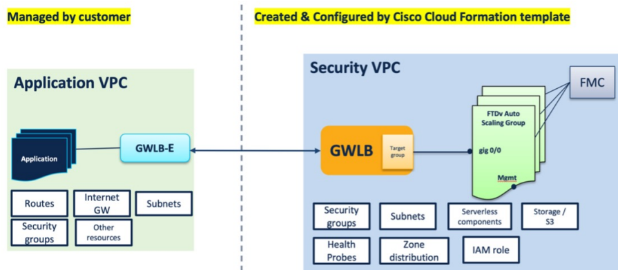
図 4 : AWS GWLB Auto Scale の導入例の図
