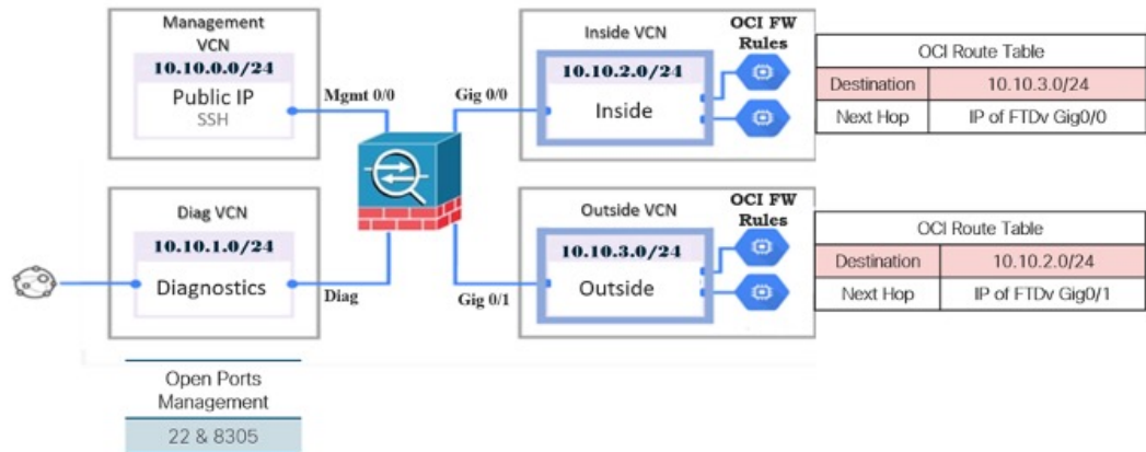
図 34 : OCI 上の Threat Defense Virtual の展開例
