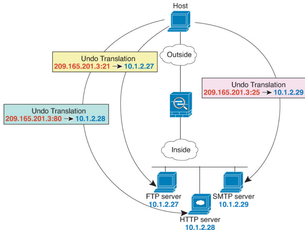
図 21: ポート変換を設定したスタティック NAT
