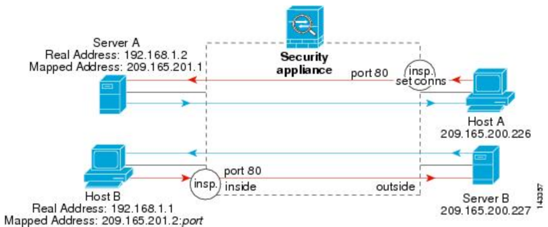
図 39: 特定のサーバーに対する HTTP インスペクションと接続制限値
