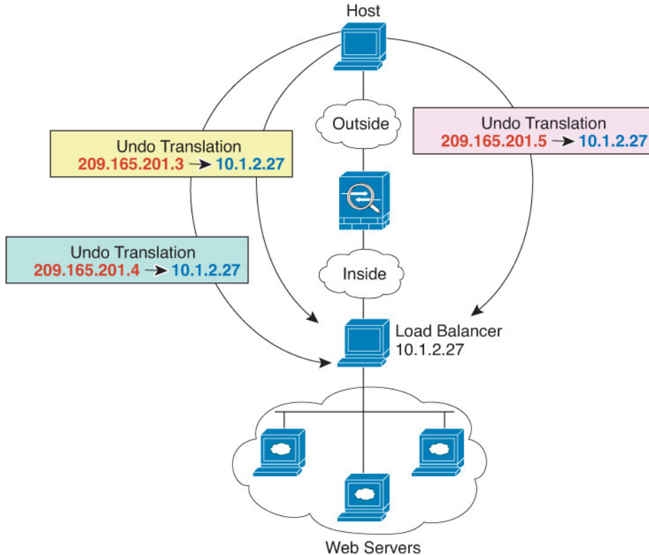
図 14: 1対多のスタティック NAT の例
