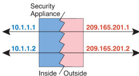
図 11:スタティック NAT
