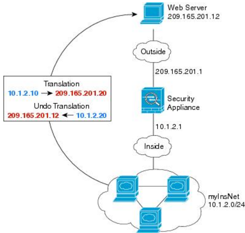
図 19: 内部の動的 NAT、外部 Web サーバーの静的 NAT
