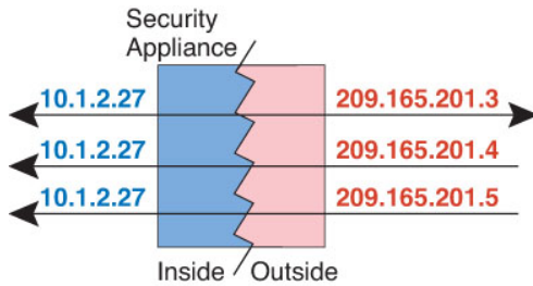
図 13: 1対多のスタティック NAT
