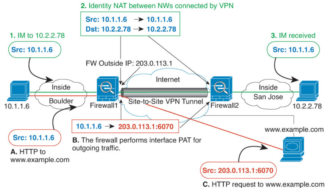
図 31: サイトツーサイト VPN のためのインターフェイス PAT およびアイデンティティ NAT
