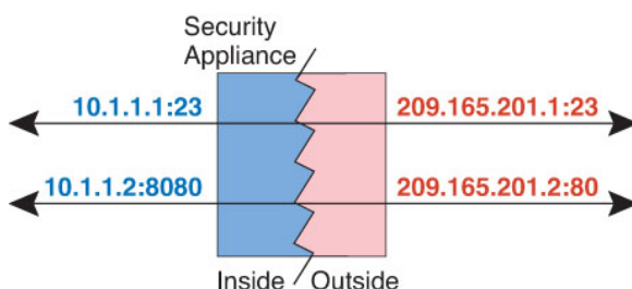
図 12:ポート変換を設定したスタティック NAT の一般的なシナリオ
